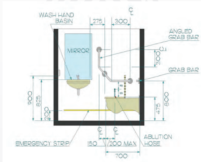
شكل ١٠٤: كشك المراض سهل الوصول.
