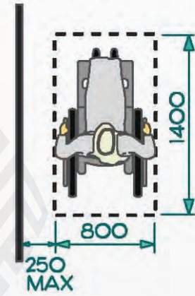
شكل ٣٤: متناول يد جانبي - المسافة القصوى للكرسي المتحرك.
