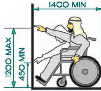
شكل ٣٢: متناول يد أمامي.
