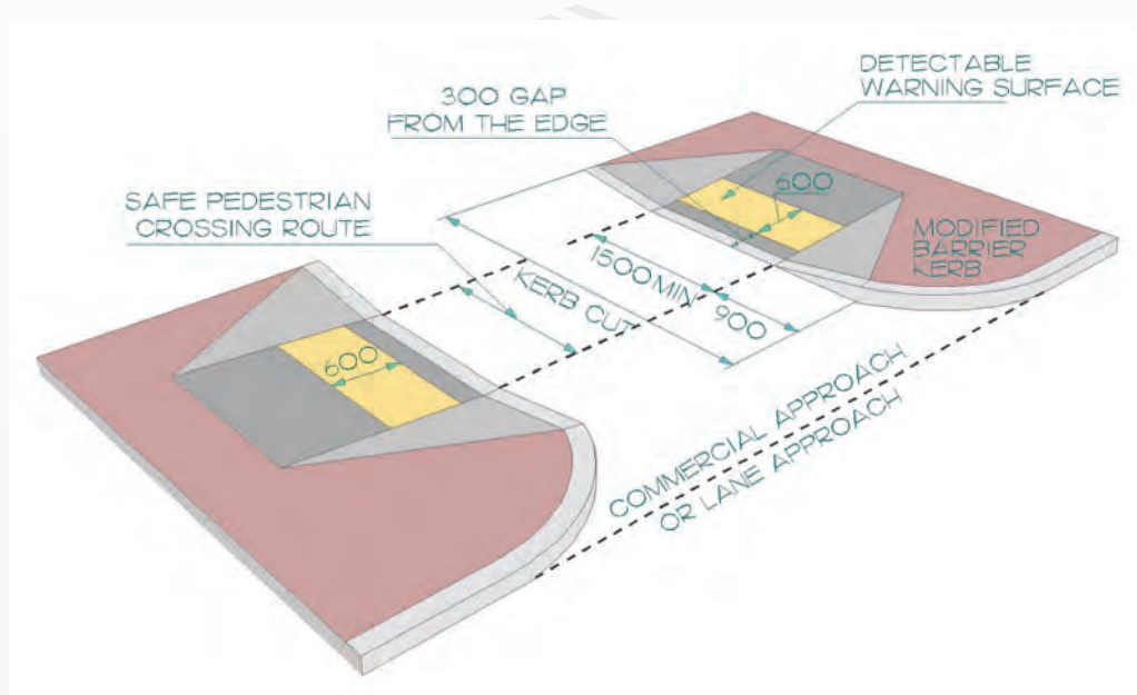
شكل و: تركيب منحدر الرصيف النموذجي.
