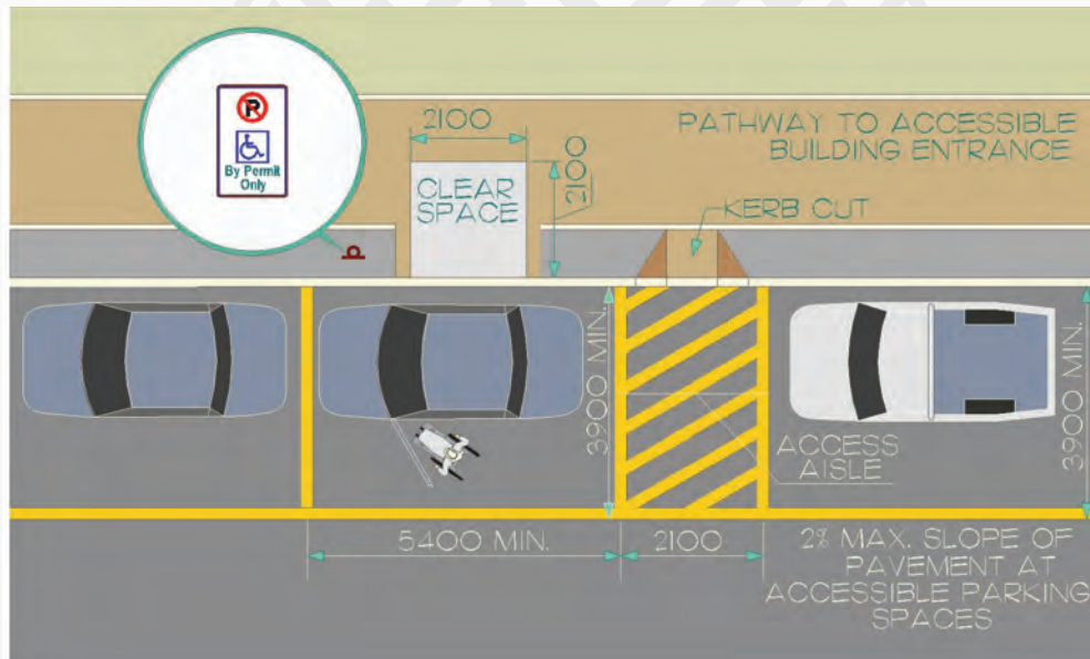
شكل ١٤٠: مناطق وقوف المركبات المتوازية.
