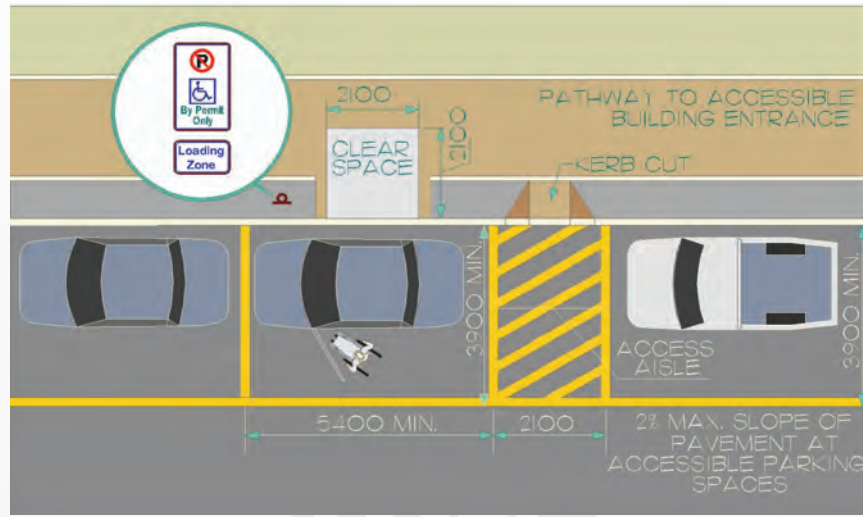
شكل ١٤٥: منطقة تحميل الركاب في الشارع.
