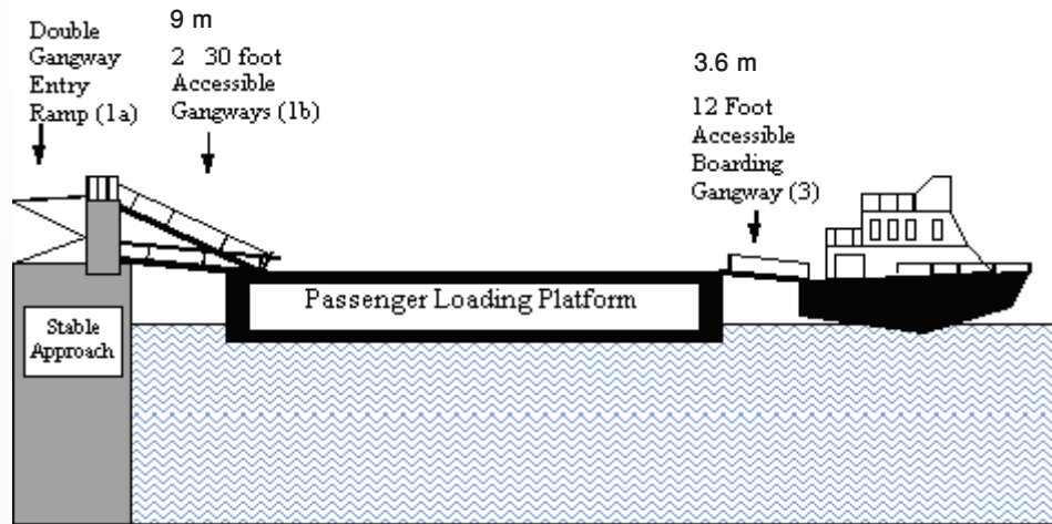
شكل ١٧٥: حل «عالي الوصول» ومكوناته (أ) و (ب) و (٣).
