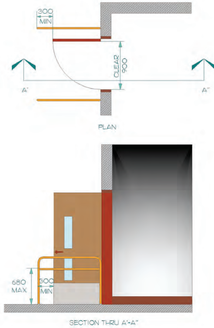
شكل ٨٣: الحواجز القابلة للكشف.
