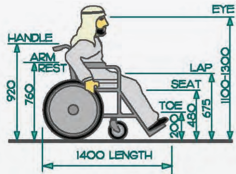
شكل ٣٦: الأبعاد النموذجية لكرسي متحرك يدوي خاص بالبالغين.
