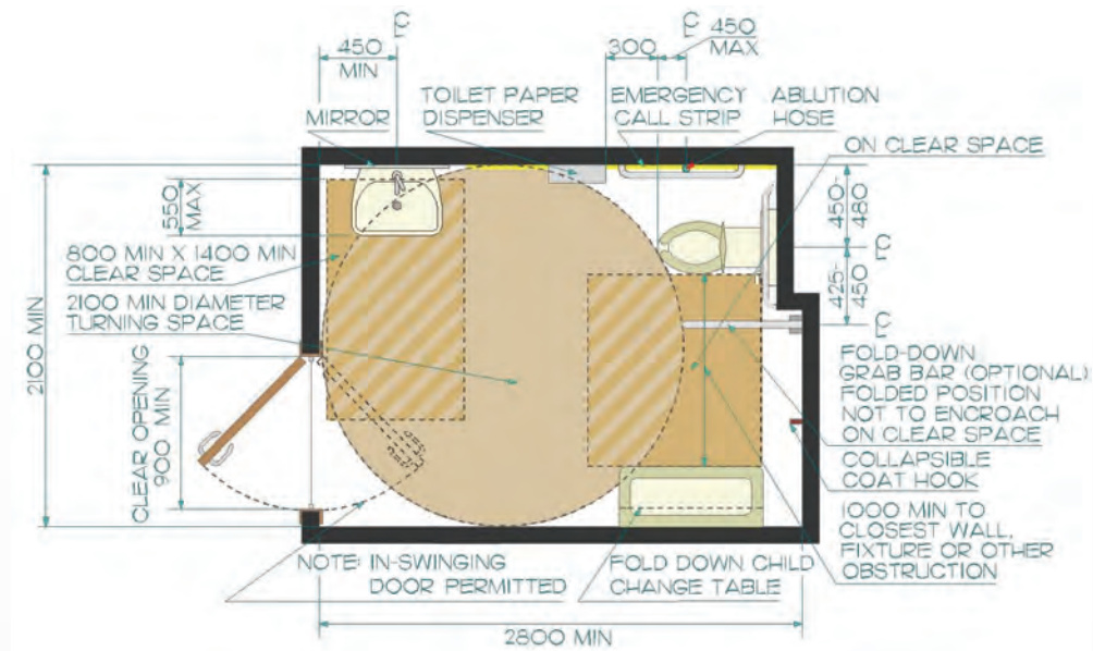
شكل ١٠٥: المرحاض الملائم لاستخدام الجنسين.
