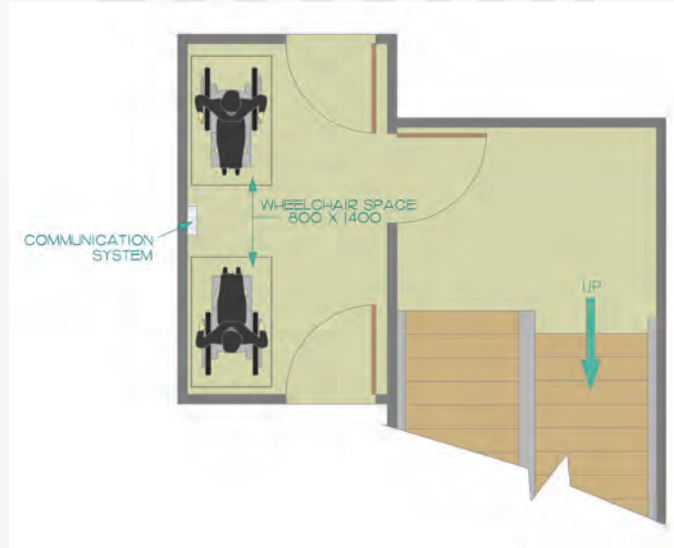
شكل ١٢٧: الرواق المحمي كم منطقة مساعدة الإنقاذ.
