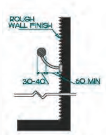
شكل ٧١: درابزين عند حائط خشن.
