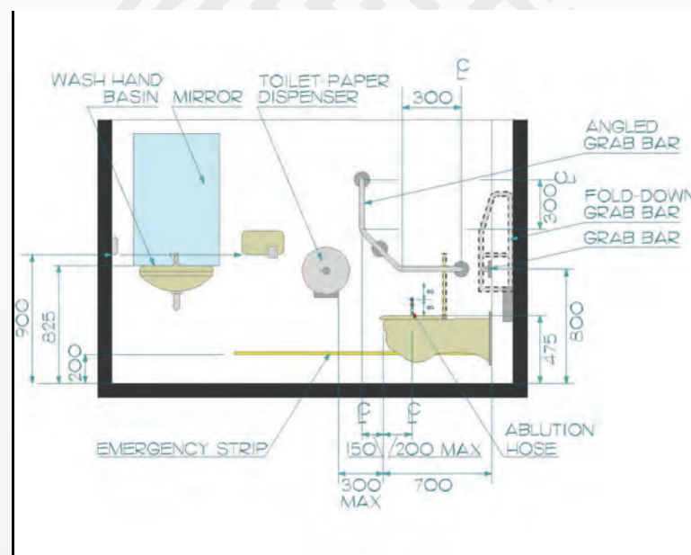
شكل ١٠٦: المرحاض الملائم لاستخدام الجنسين.
