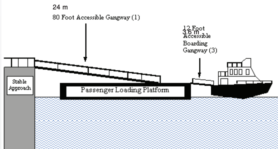
شكل ١٧٦: حل عالي الوصول أو منخفض الوصول ذو مكونات (١) و (٣).
