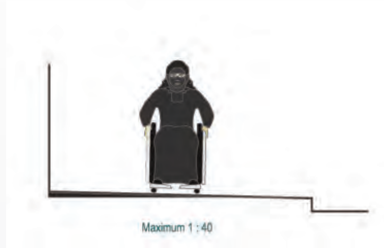
شكل ١٣٢: أقل أبعاد لتخطيط / تصميم الطريق المائل.
