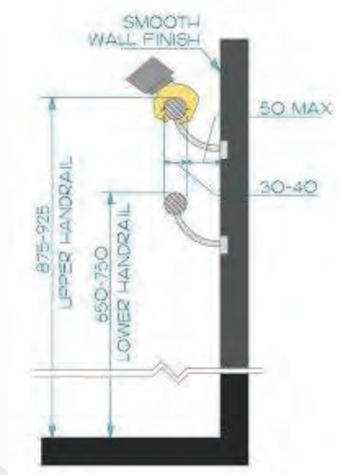
شكل ٧٠: ارتفاع وتركيب الدرابزين.
