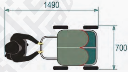
شكل ٤١: مساحة أرضية خالية من العوائق لعربة يد مزدوجة متجاورة.
