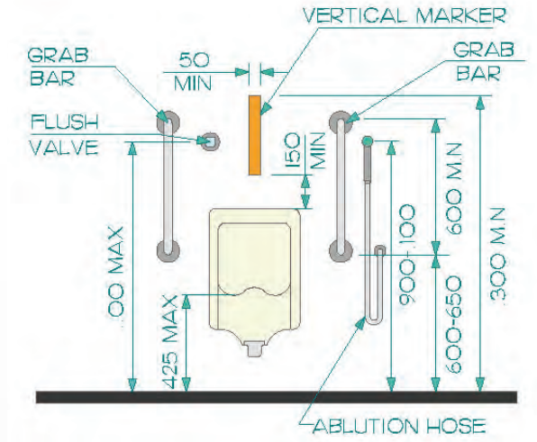
شكل ١١٧: ارتفاع مرحاض التبول. جميع الأبعاد بالمليمتر ما لم يذكر غير ذلك.
