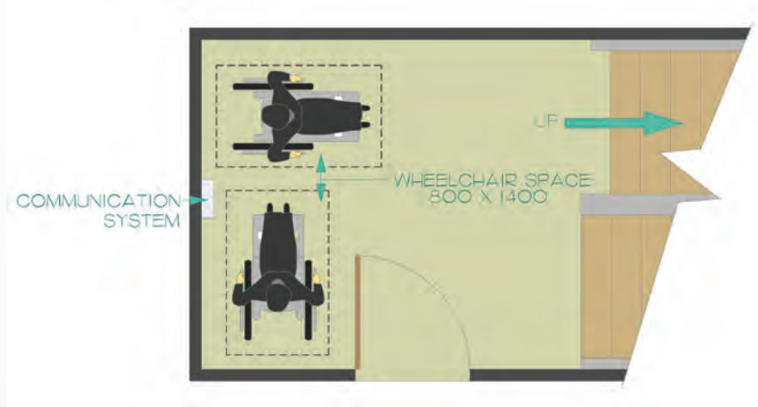
شكل ١٢٦: منطقة الهبوط زائدة الحجم كم منطقة مساعدة الإنقاذ.
