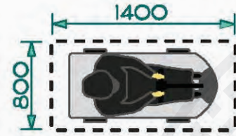
شكل ٢٣: مساحة أرضية خالية لشخص يستخدم سكوتر التقل.
