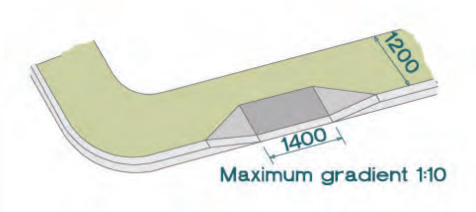
شكل ١٣١: أقل قدر من متطلبات أبعاد منحدر الرصيف.
