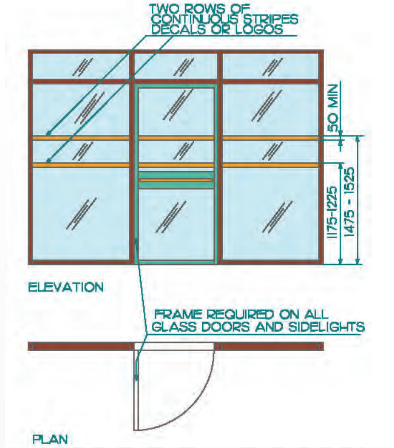
شكل ٨٦: علامات الأبواب المزججة بالكامل، النوافذ الجانبية ولوحات الرؤية. كل الأبعاد بالمليمتر إذا لم يذكر غير ذلك.
